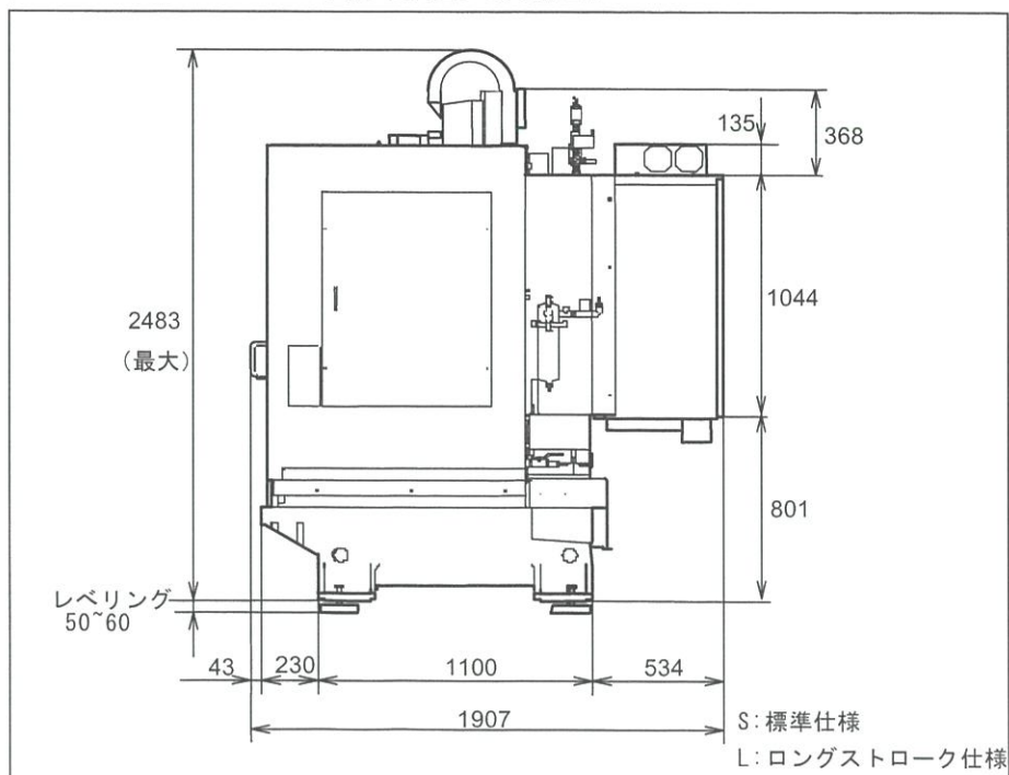
図2-4 TC-S2B外觀寸法図（右側面）
